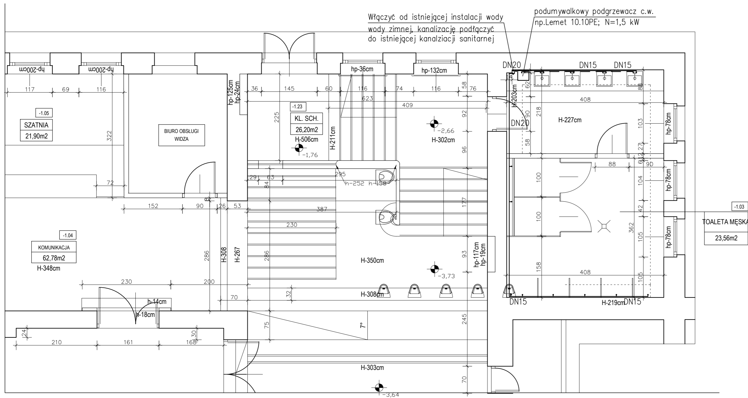
RZUT PIWNIC – WOD-KAN i C.W.
